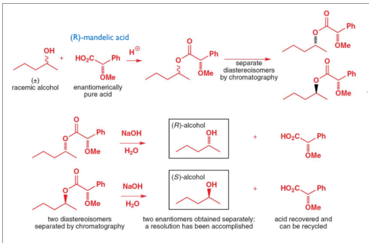
Figura 14: Esempio di utilizzo di un resolving agent .
