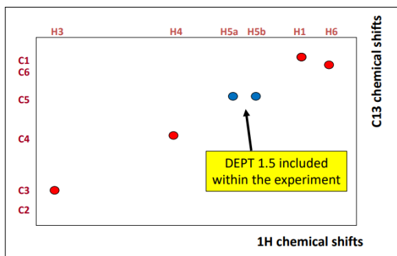
Figura 54: Rappresentazione ideale di uno spettro HSQC
