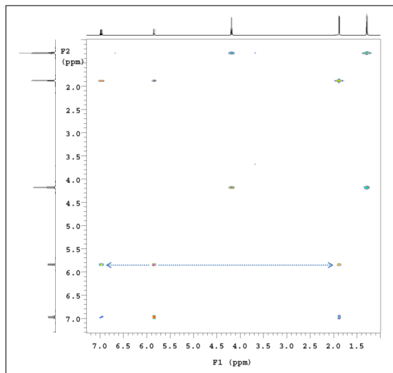
Figura 51: Spettro COSY dell'etil(E)-butan-2-ato
